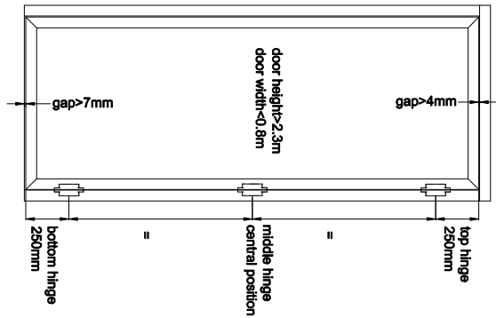
Over-height Door
