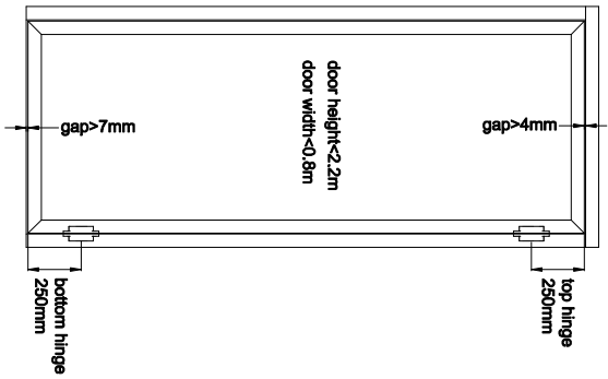
Normal Door
