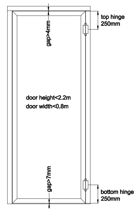
Normal Door
