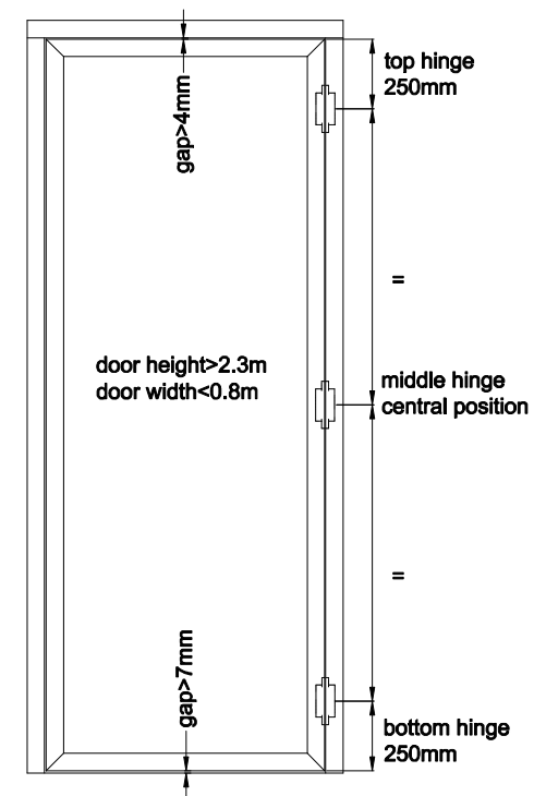
Over-height Door
