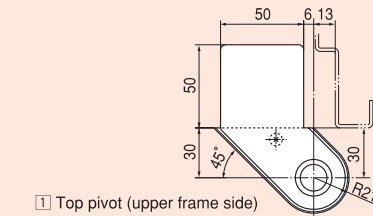
1 Top pivot (upper frame side)
