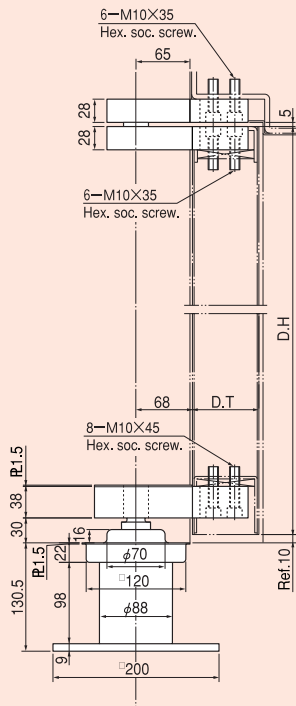
2 Top pivot (door side)
